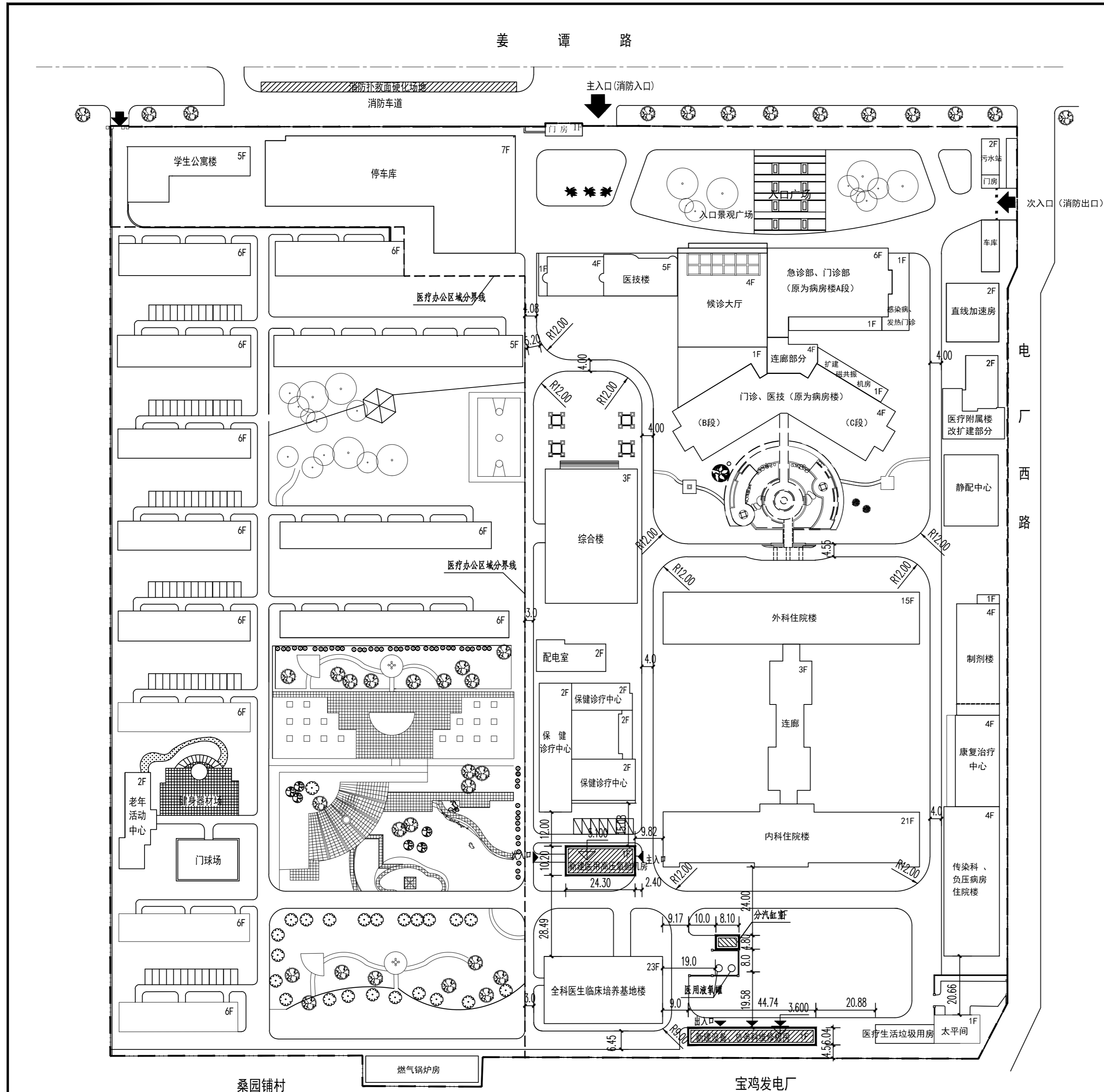
总平面图 1:1000
