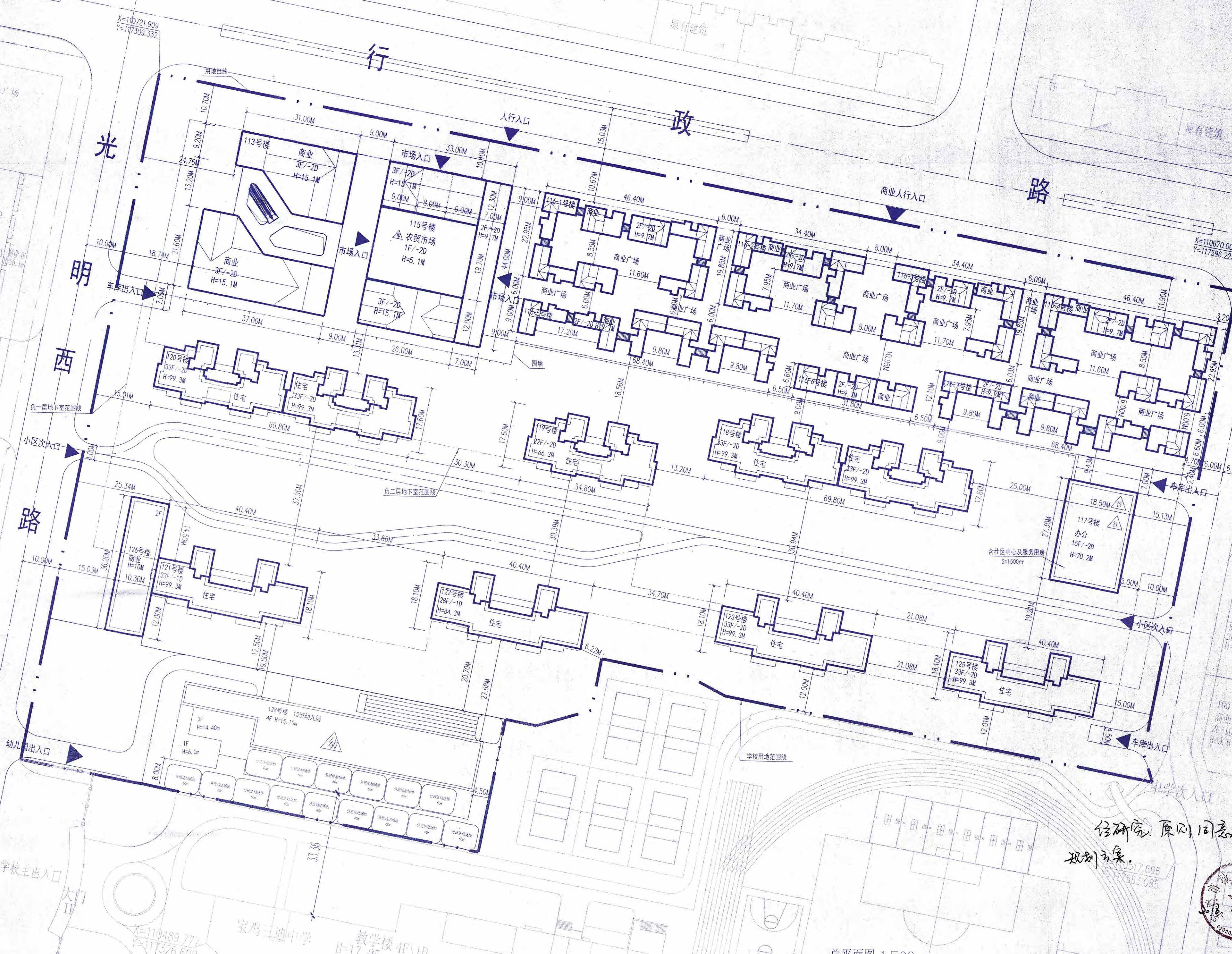
总平面图 1:500
